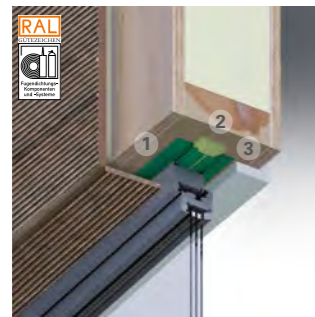
1 Fugendichtungsfolie mit Fensterfolienkleber 2 Schaum
