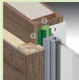
1 Fugendichtungsfolie mit Fensterfolienkleber 2 Schaum 3 Fugendichtungsband
