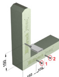
Doppelverschraubung
