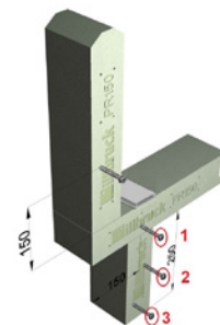
Einfachverschraubung mit Stützklötz
