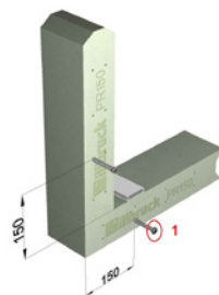
Einfachverschraubung
