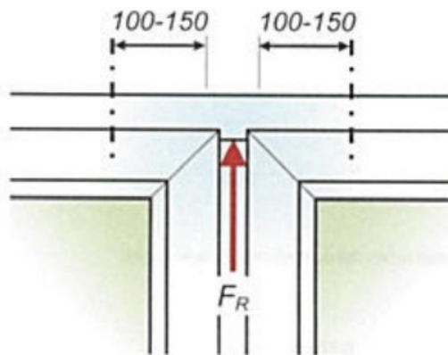
Doppelbefestigung symmetrisch
