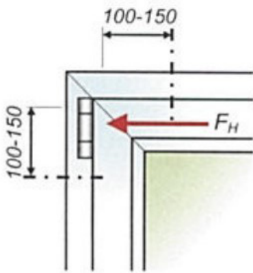
Über-Eck-Befestigung
