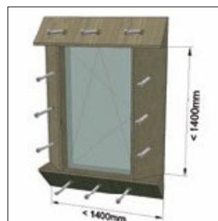
Obr. 5: Sicherungsschrauben 1 fig. špára 10 mm
