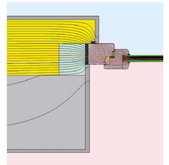
Günstigerer Isothermenverlauf
