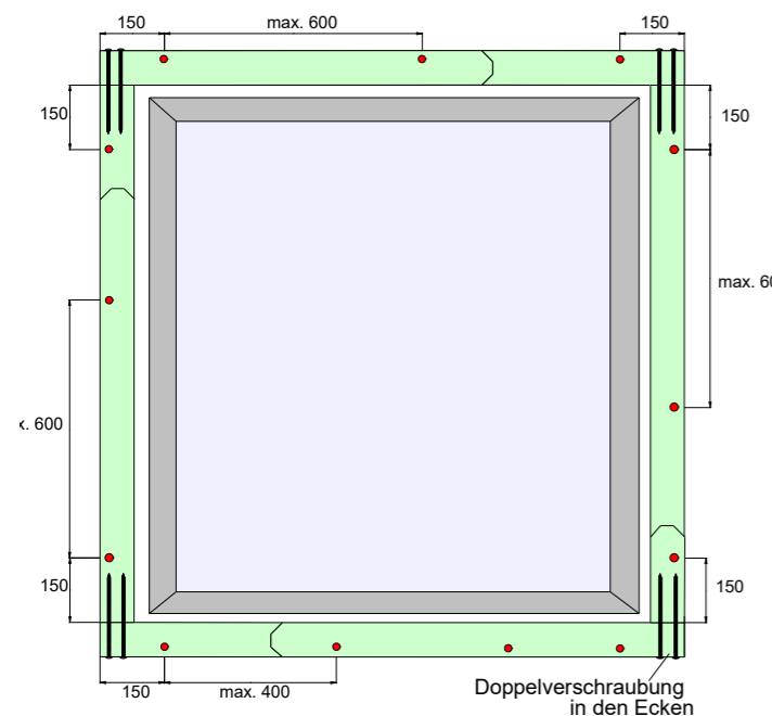
Schraubschema RC2, Schraubabstand bei RC3 250 mm und Eckverschraubung
